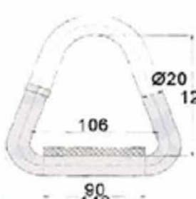
LDR105-20106
