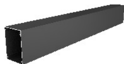
名称: 立柱/横梁 尺寸: 90*125*2 材质: 6063-T5
